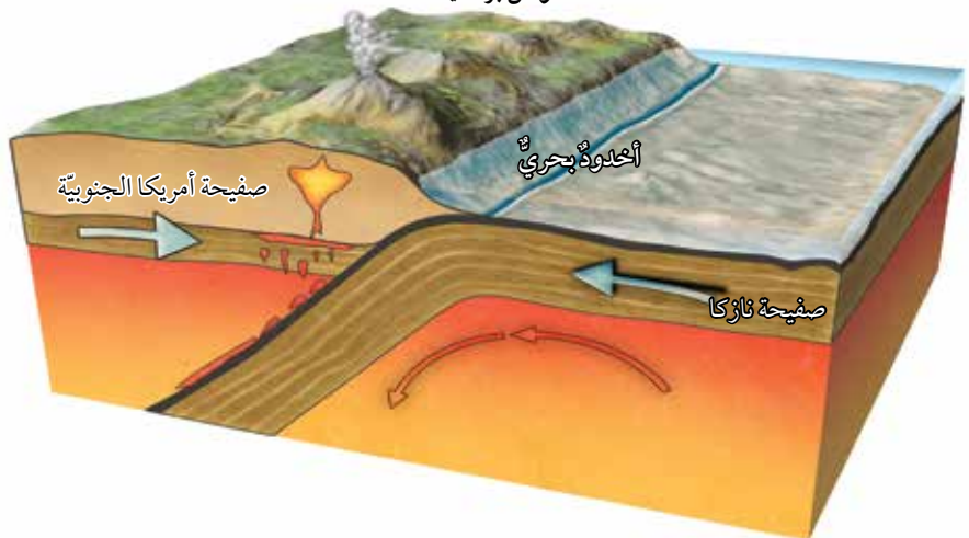
أفواس بركانية
