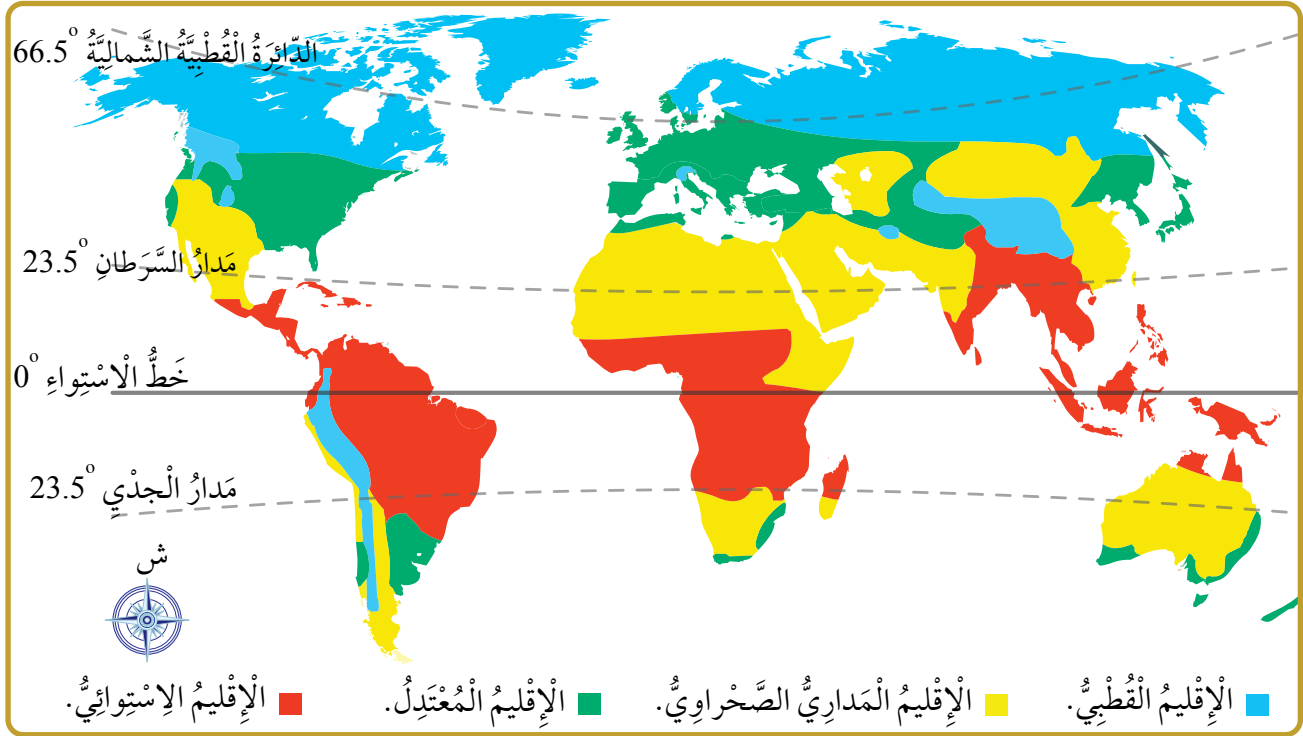
الشكل (15): الأقاليم المناخية الرئيسة في العالم.
