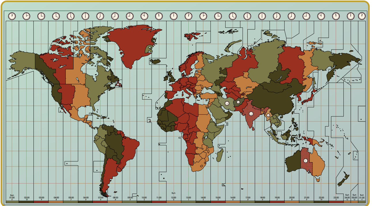
الشَّكْلُ (1): الْمَنَاطِقُ الزَّمَنِيَّةُ فِي الْعَالَمِ.
